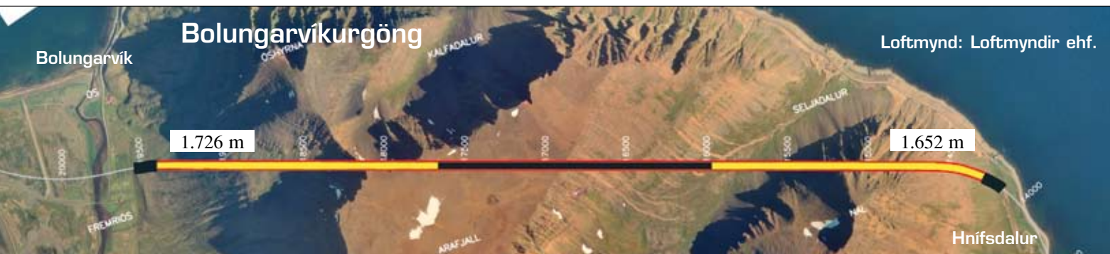
Bolungarvíkurgöng 18. maí. Gröftur gekk vel í viku 20. Frá Hnífsdal voru sprengdir 53 m og er heildarlengd þeim megin 1.652 m. Frá Bolungarvík voru sprengdir 55 m og er heildarlengd þeim megin 1.726 m. Samtals er því búið að sprengja 3.378 m eða tæp 65,5% af heildarlengd.
